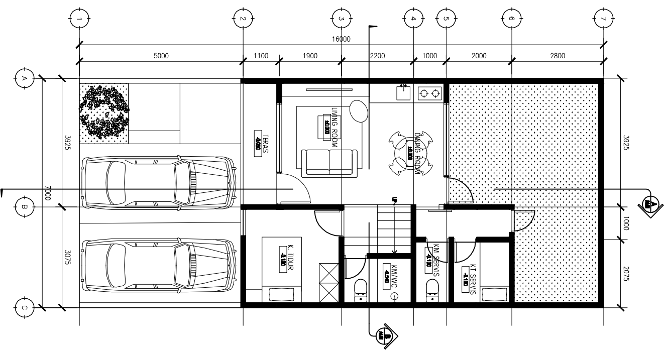
1 DENAH L.T. DASAR A2-1 1:100
