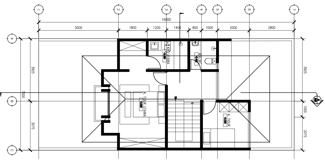
1 DENAH L.T. ATAS A2-1 1:100
